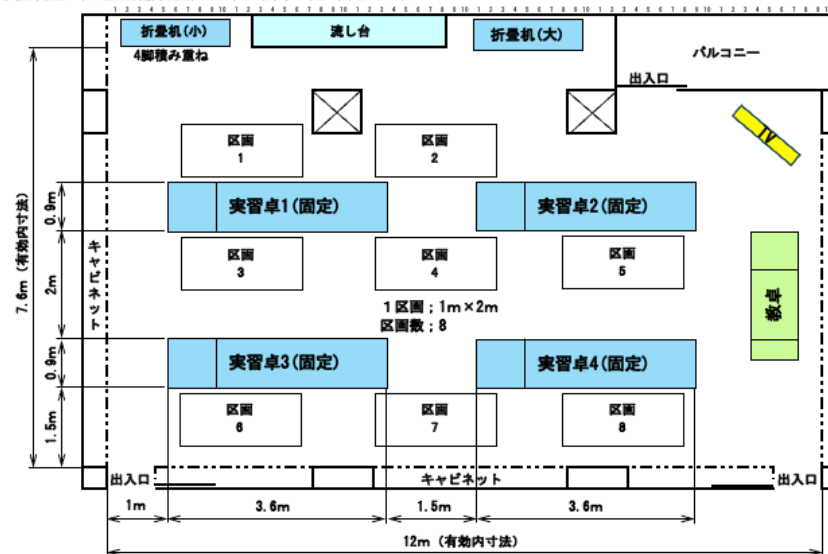
家庭科室（女性配慮者室）基本区割り（感染症対応）
